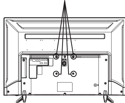
壁掛け金具取り付け用ネジ穴
